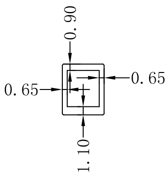
壁厚示意图
